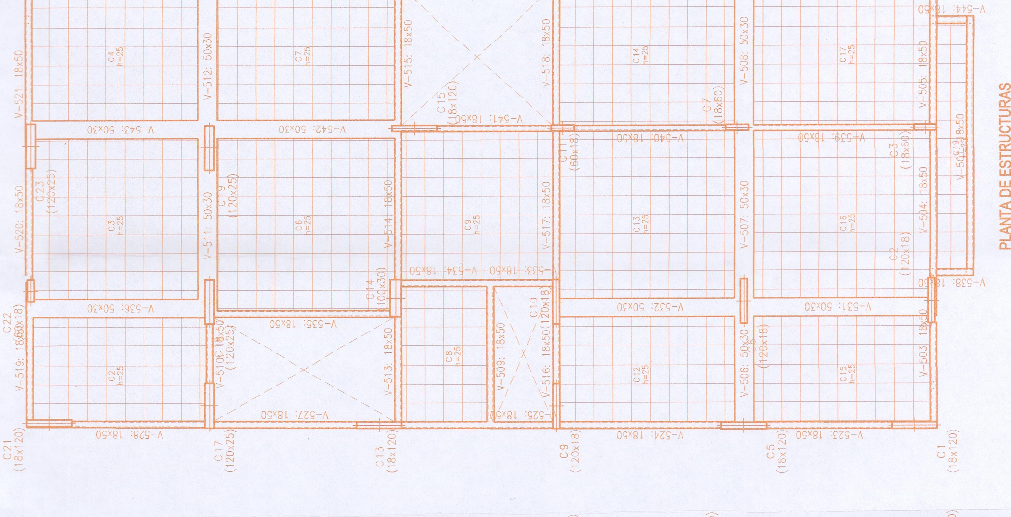
PLANTA DE ESTRUCTURAS Sobre PISO 3
