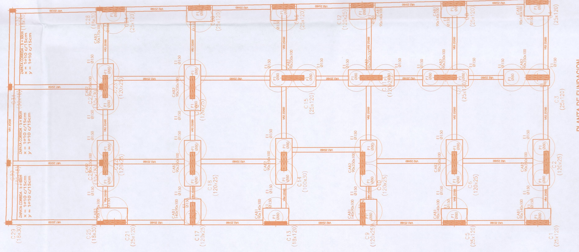
PLANTA DE FUNDACION Sobre SUELO Escala: 1:100
